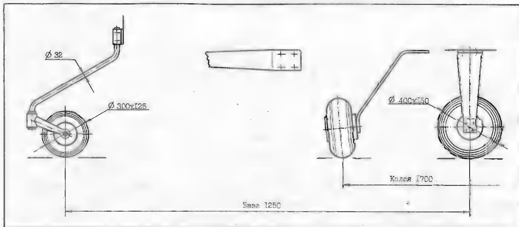
Рис. 2. Шасси самолета «Гельфин». Материал стоек — Сталь 65 Г.
